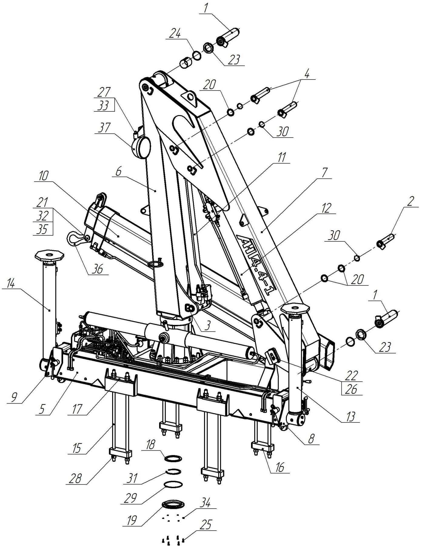
Рисунок 1 - Соединение основных сборочных узлов
