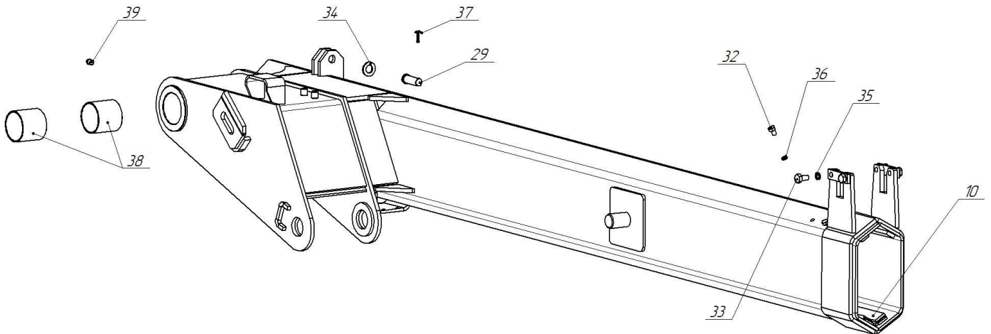
Рисунок 11 – Основная секция
