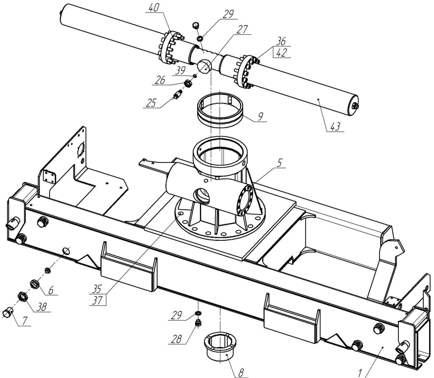
Рисунок 5 – Платформа неповоротная
