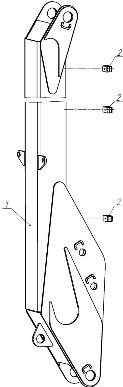
Рисунок 9 – Стрела первая
