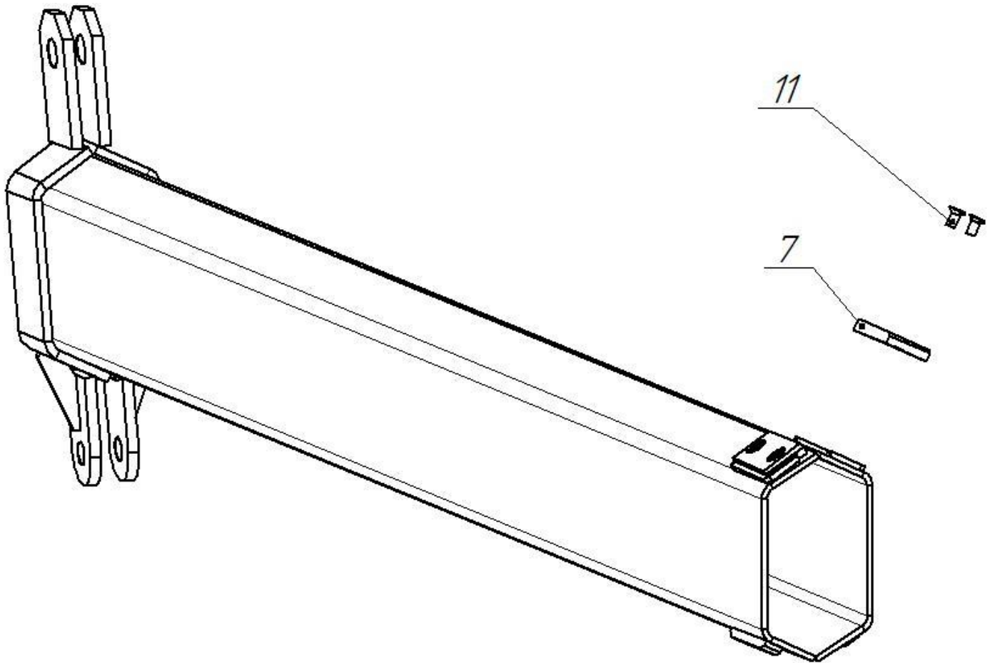
Рисунок 12 – Секция телескопическая
